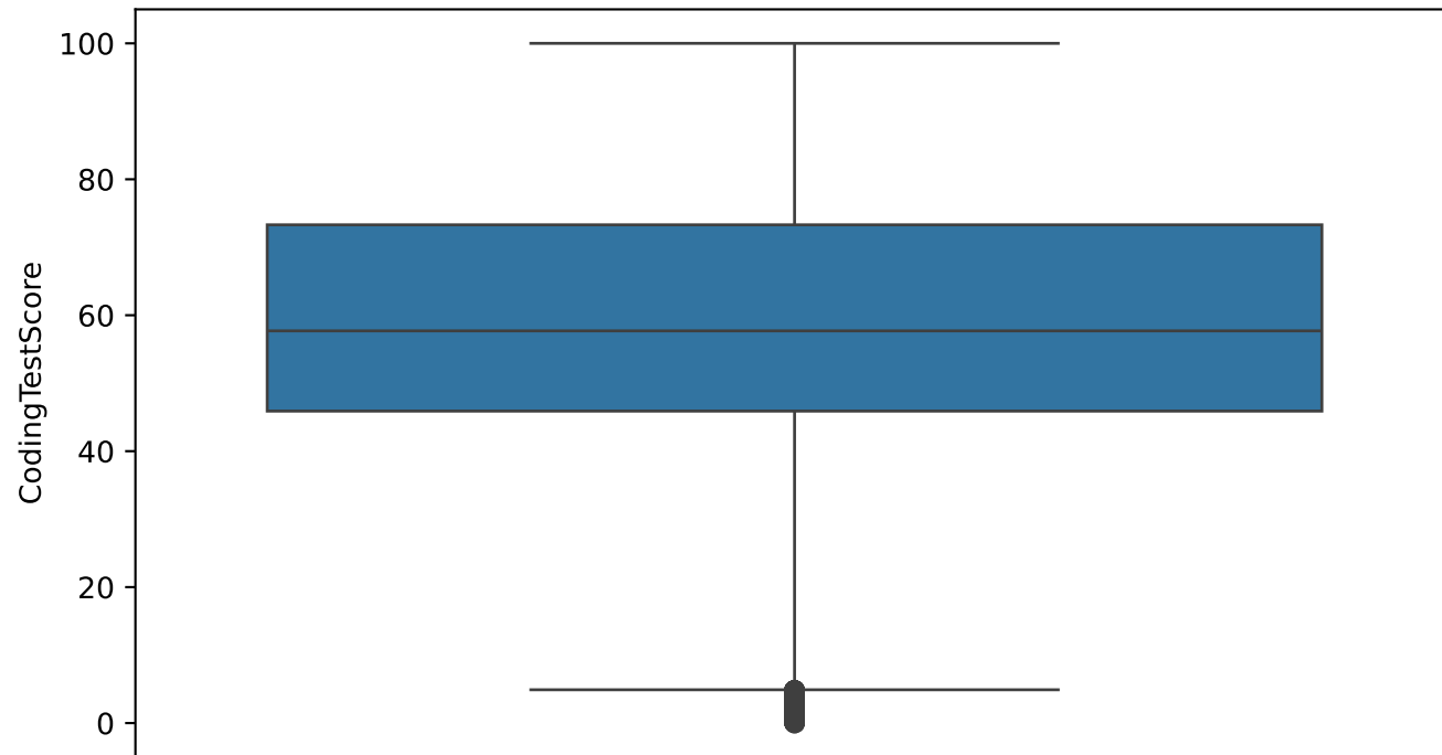
CodingTestScore
